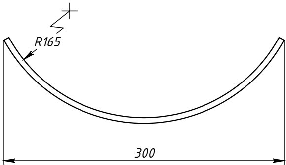
Поз.3 (Ложемент)
